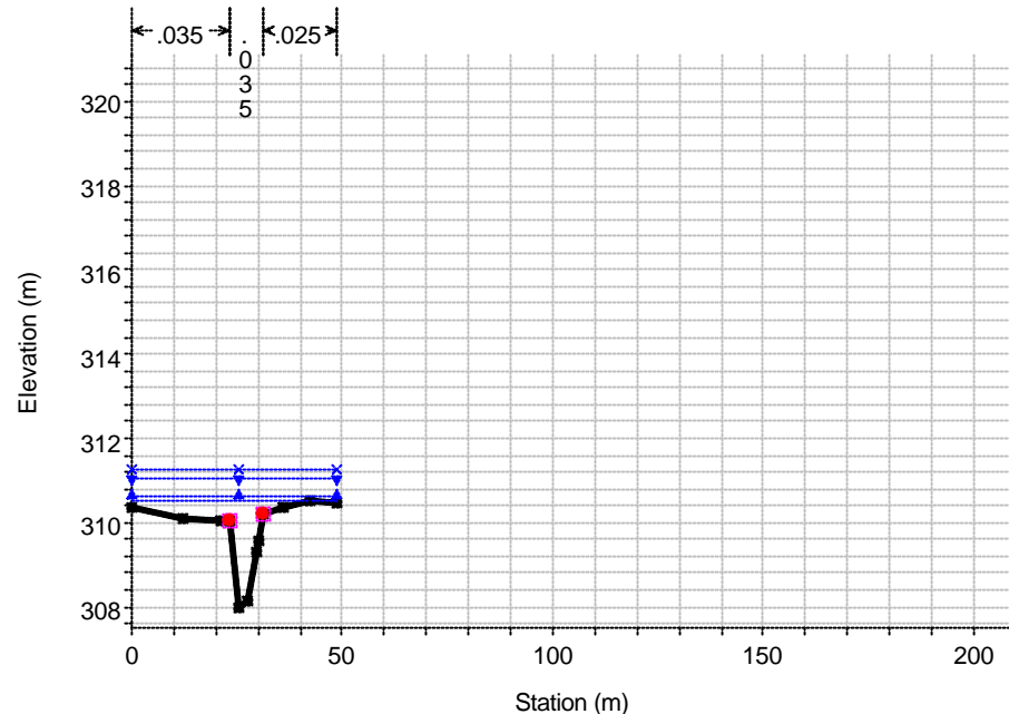
RS = 16 sez 125 Torrente Fiumicello
