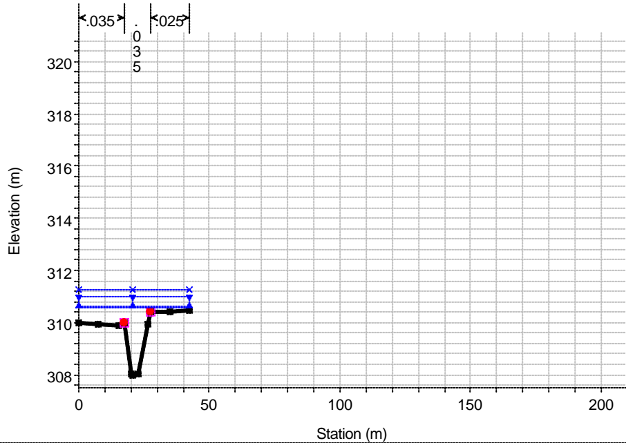
RS = 17 sez 124 Torrente Fiumicello
