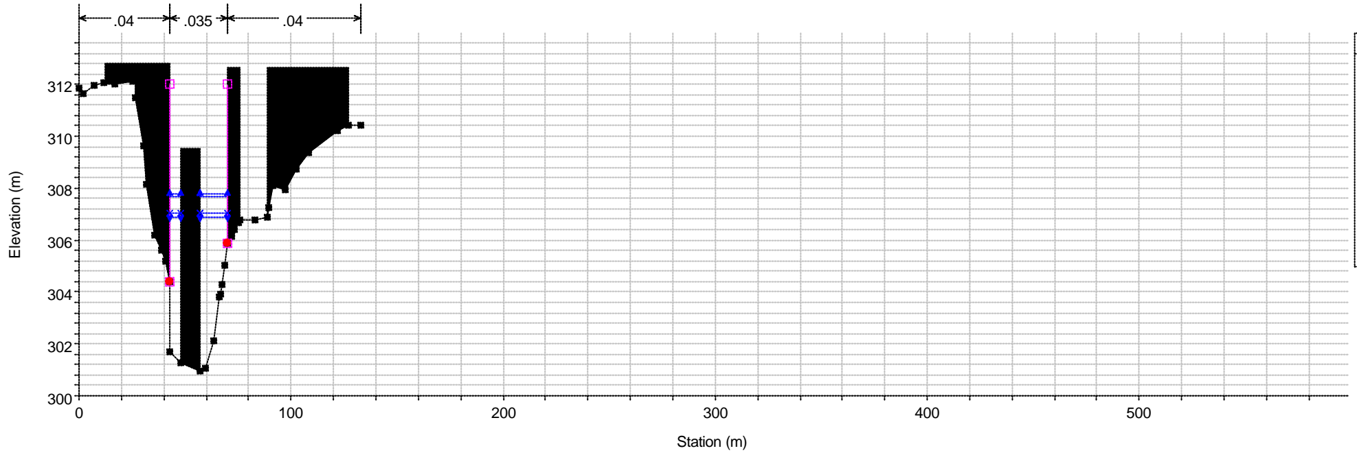
RS = 12 sez 120 monte ponte Fiume Tevere
