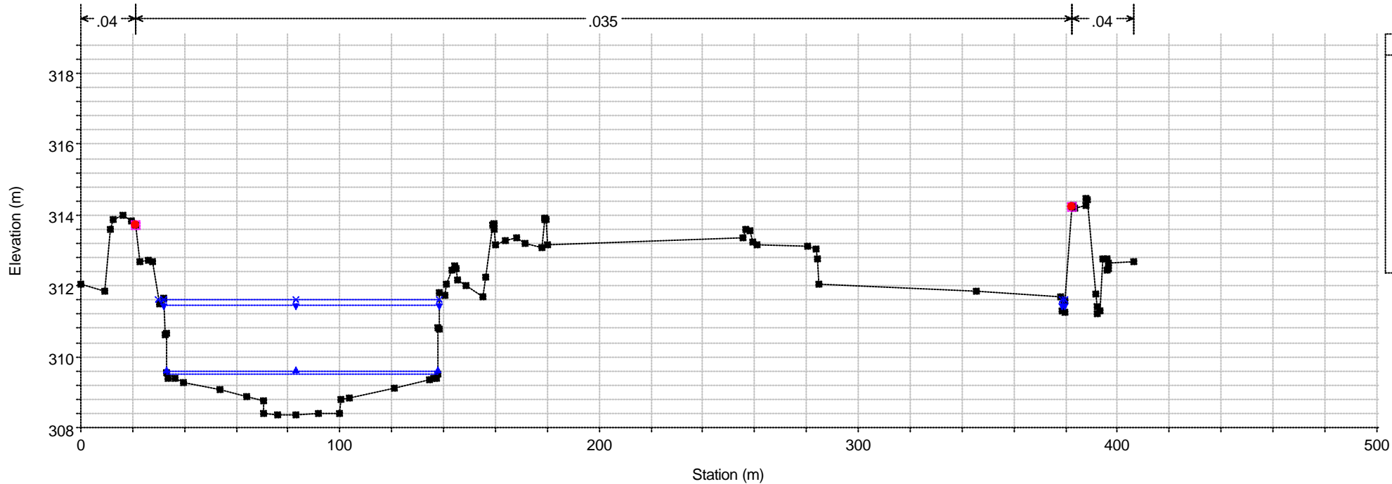
RS = 19 sez 190 Fiume Tevere
