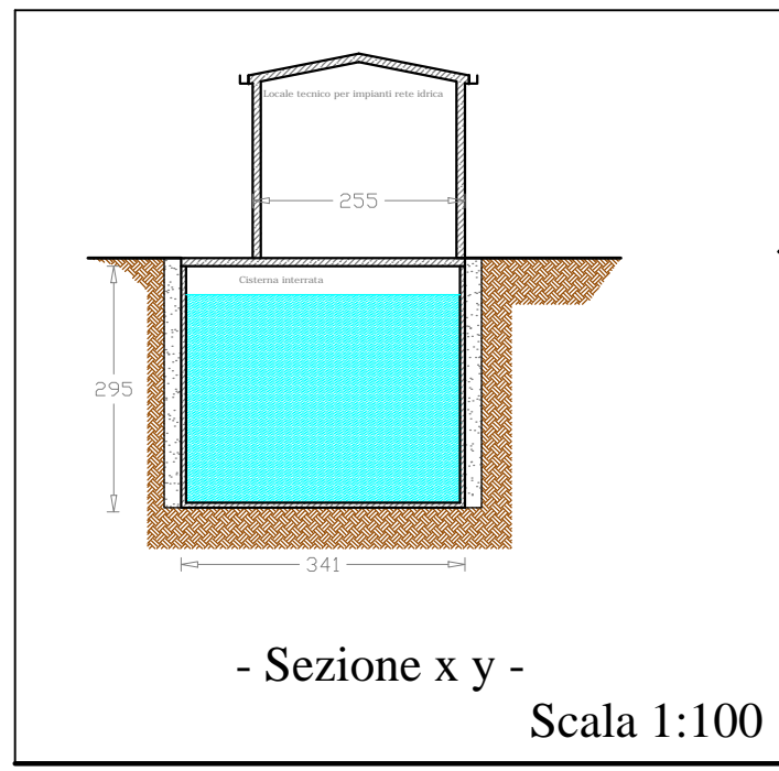
- Locale tecnico per impianti rete idrica - L255 x P260 x H235 cm
