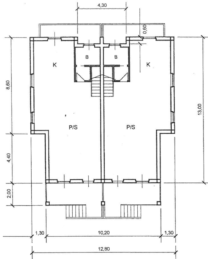
PIANTA PIANO RIALZATO
